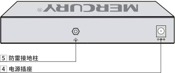
图 2-8 SE106P 后面板示意图
