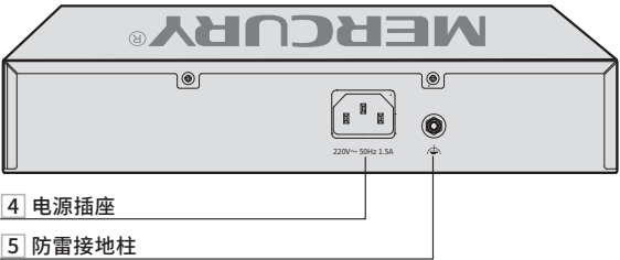
图 2-7 SE109P 后面板示意图
