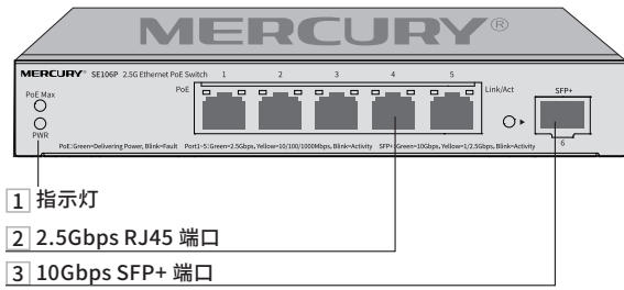
图 2-4 SE106P 前面板示意图
