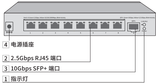
图2-5 SE109后面板示意图
