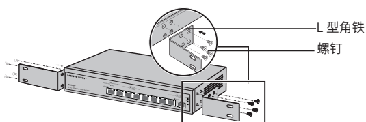
图 3-2 角铁安装示意图
